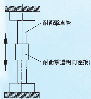
管體與接頭接合伸延試驗機
